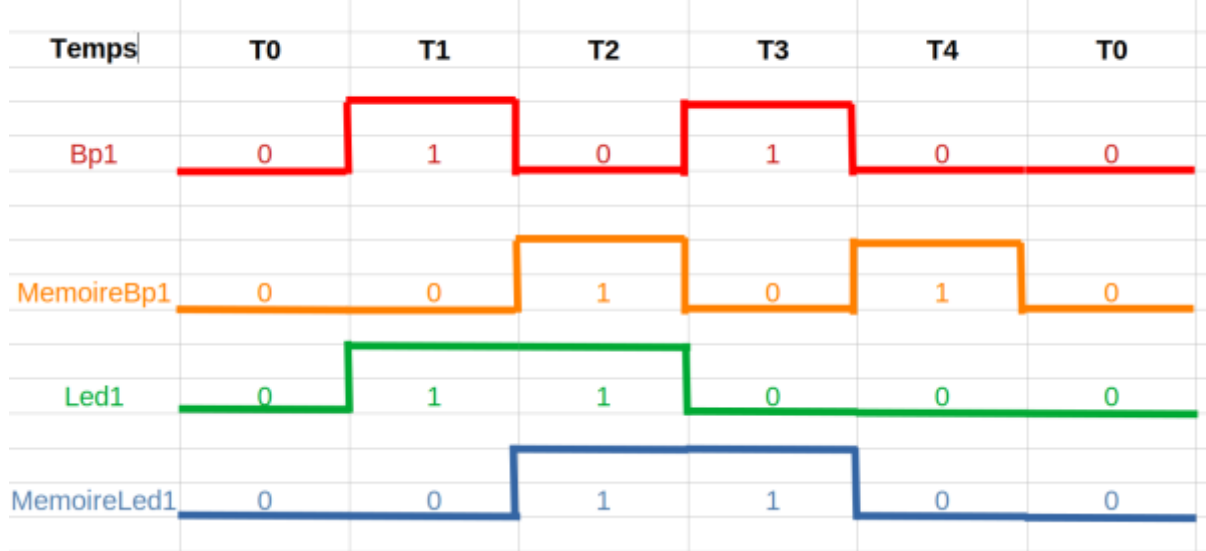
diagramme Bouton poussoir en interrupteur sans clignotement
