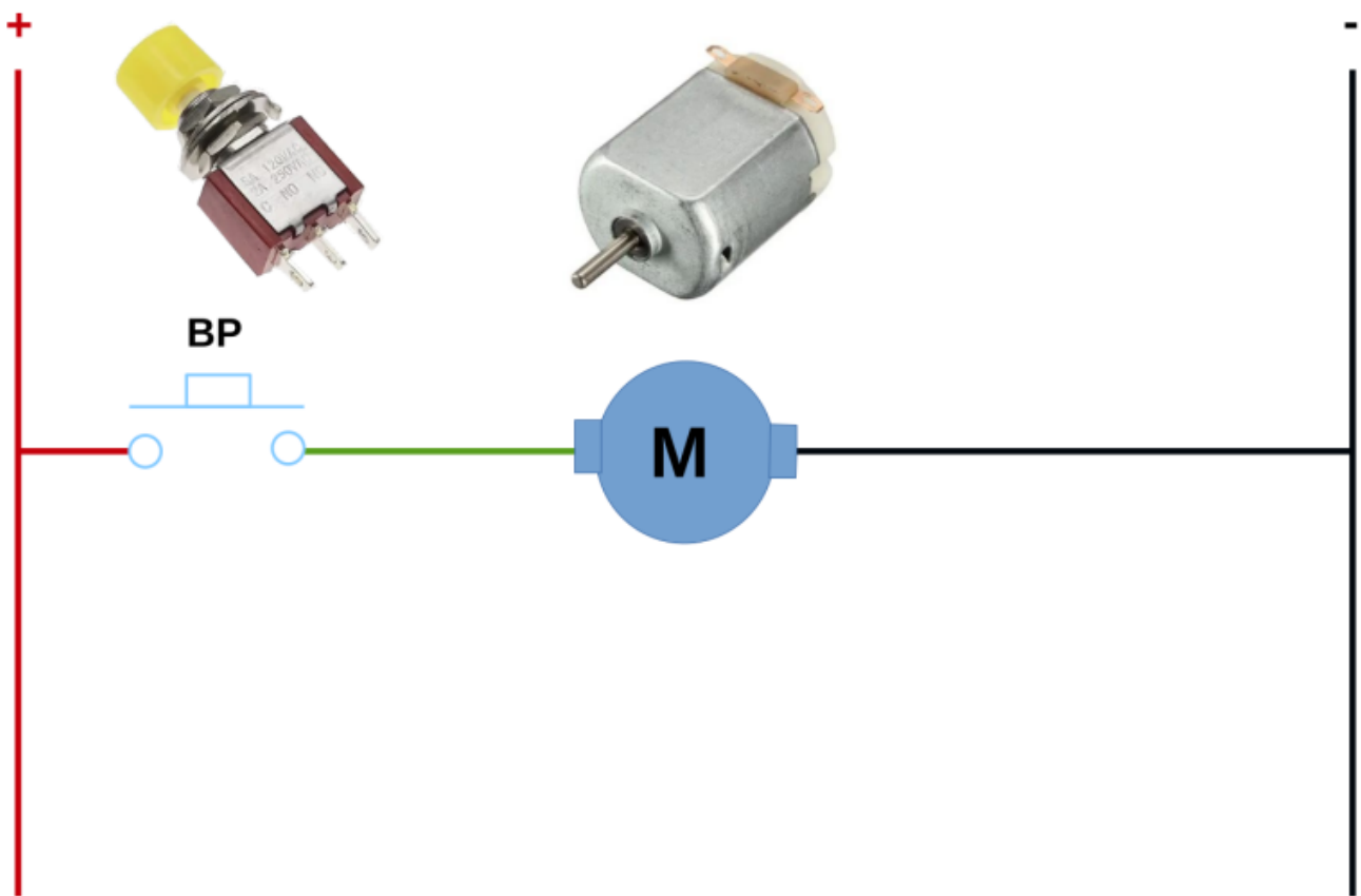
Interrupteur Double 2 sens moteur
