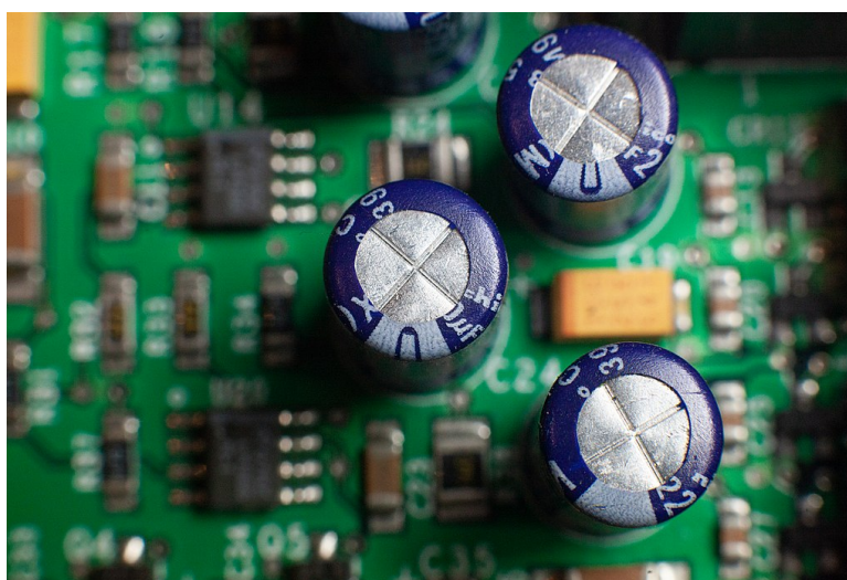
Condensateurs chimiques en bon état
